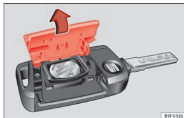
Fig. 134 Chiave del veicolo: aprire il coperchio del vano della batteria.
