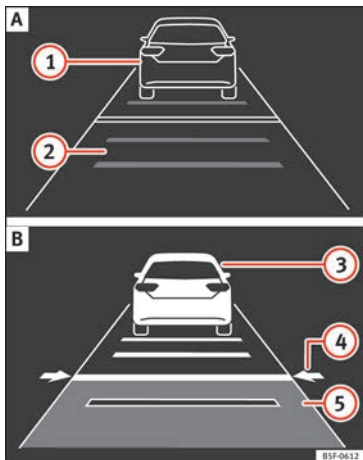
Fig. 202 Sul display del quadro strumenti: (A) ACC temporaneamente inattivo, rilevamento veicolo precedente, distanza temporale regolata. (B) ACC attivo, rilevamento veicolo precedente, viene regolata una distanza temporale.
