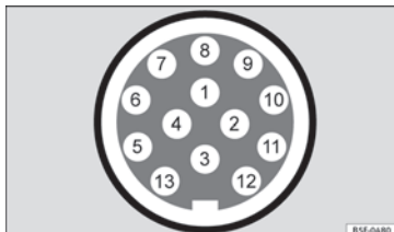
Fig. 243 Rappresentazione schematica: assegnazione dei pin della presa di corrente del rimorchio.
