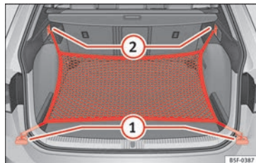
Fig. 179 Nel bagagliaio: occhielli ① e ganci ② per agganciare la tasca a rete (modello LEON ST).
