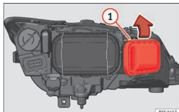
Fig. 105 Lampadina dell'indicatore di direzione.
