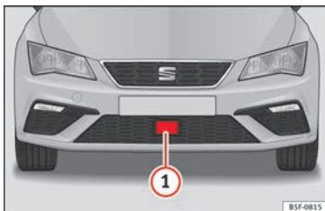
Fig. 203 Sul paraurti anteriore: sensore radar.
