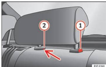
Fig. 147 Poggiatesta per il sedile posteriore centrale: punto di sblocco.
