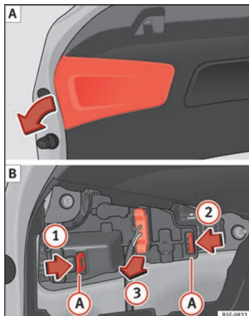
Fig. 113 Rimuovere la copertura nel portellone e smontare il portalampe.
