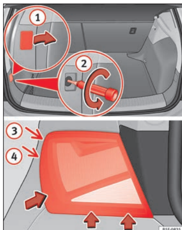
Fig. 111 Bagagliaio: posizione della vite di fissaggio del fanale di coda. Smontaggio del fanale di coda esterno.
