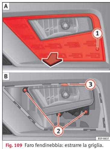
Fig. 109 Faro fendinebbia: estrarre la griglia.
