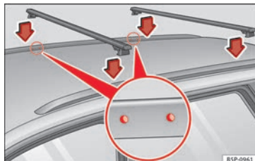
Fig. 185 LEON ST: punti di fissaggio delle barre longitudinali per il portapacchi da tetto.
