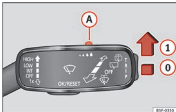
Fig. 144 Leva dell'impianto tergicristalli Regolazione del sensore pioggia A .
